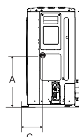
8/10/12/14/16 kW (jednotka:mm)
