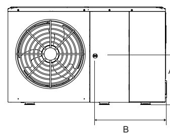
8/10/12/14/16 kW (jednotka:mm)
