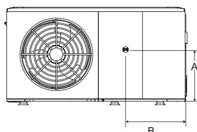
4/6 kW (jednotka:mm)
