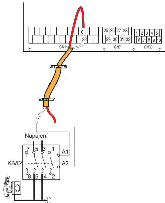
Venkovní oběhové čerpadlo P_o
